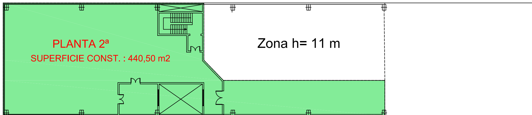
PLANTA SEGUNDA
