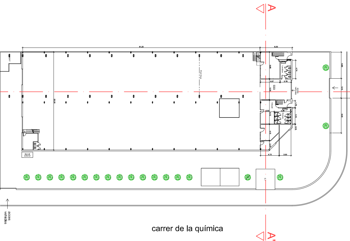
planta baixa
